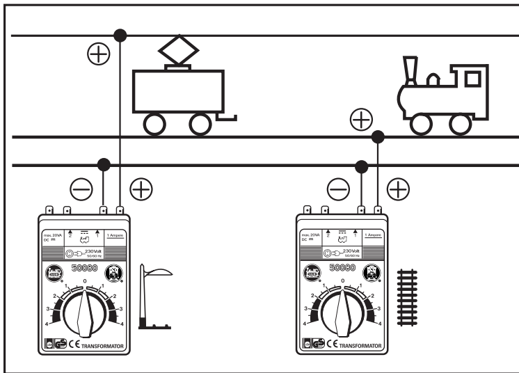
Bild 3 & 4, Oberleitungs-Betrieb Fig. 3 & 4, Catenary operation Img. 3 & 4, Fonctionnement caténaire
