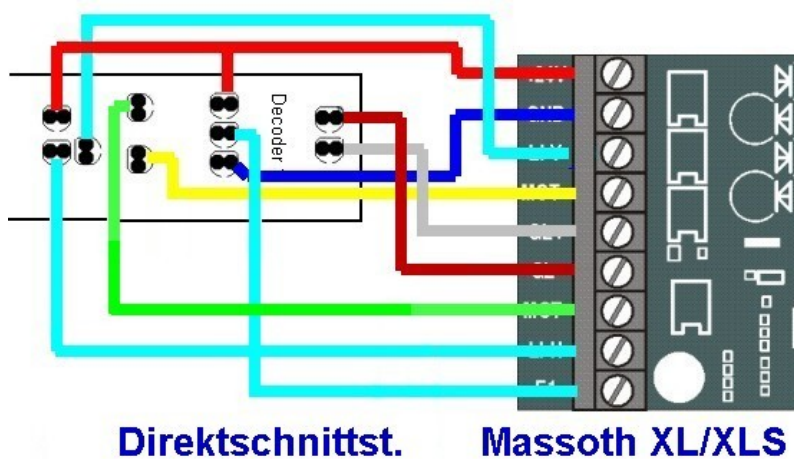
Abbildung 1: Direktschnittstelle 1
