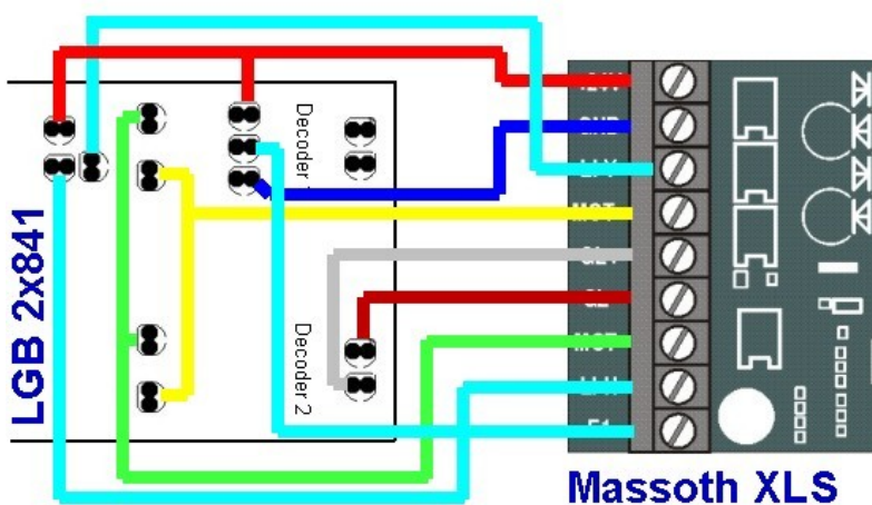
Abbildung 2: Direktschnittstelle 2
