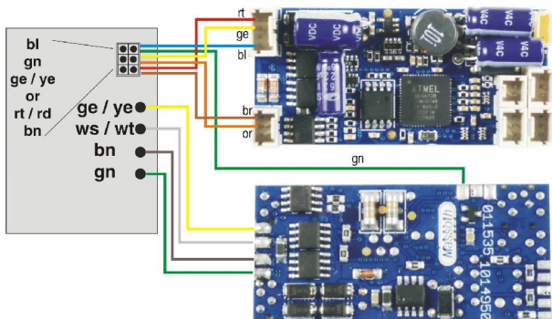
Abbildung 5: Einbau in Lok mit LGB Dekoder Schnittstelle
