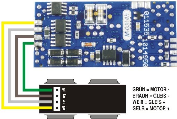
Abbildung 3: Anschluss an LGB® Getriebe
