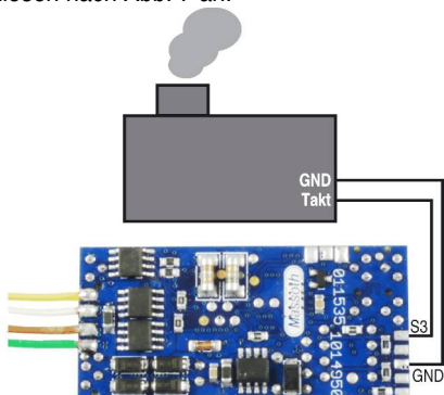
Abbildung 7: Andere gepulste Verdampfer
