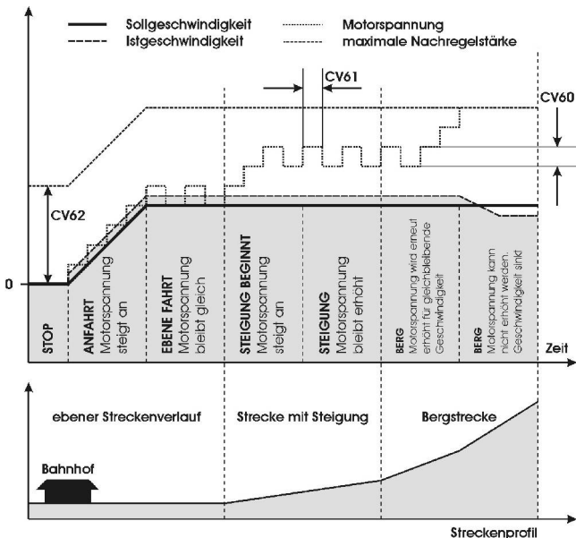
Abbildung 9: Funktionsweise der Lastregelung
