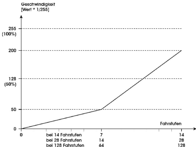
Abbildung 8: Interne Fahrkurve des eMOTION LS Sounddekoders, einstellbar über CV2 (Anfahrspannung), CV5 (Maximalgeschwindigkeit), CV6 (Mittengeschwindigkeit)
