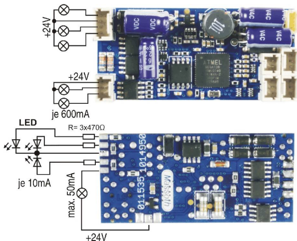
Abbildung 6: Licht und Funktionsausgänge und deren Verschaltung
