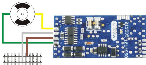
Abbildung 2: Einbau des eMOTION LS
