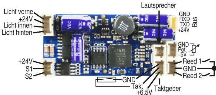
Abbildung 1: Belegung der Anschlussbuchsen
