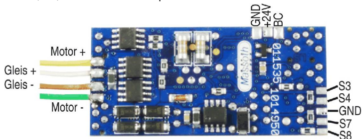
Abbildung 4: Belegung der Anschlusslötkontakte (Unterseite)
