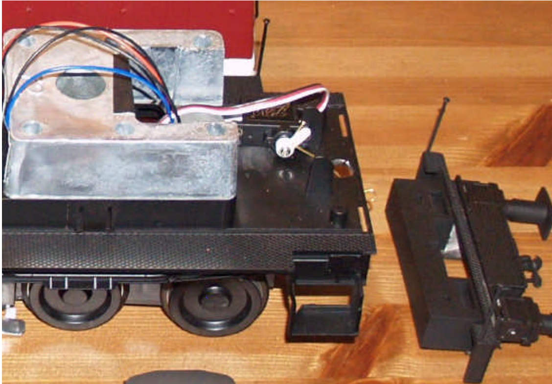
Beispiel für Servo einbau
